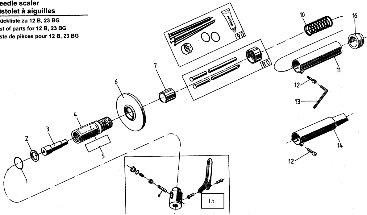
Onderdelenlijst Naaldenbikhamers 12B
